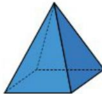
pirámide
