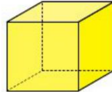
cubo
