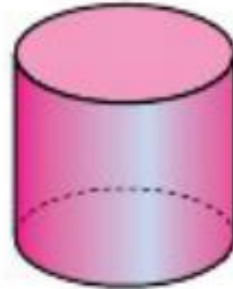
cilindro
