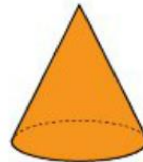
cono
